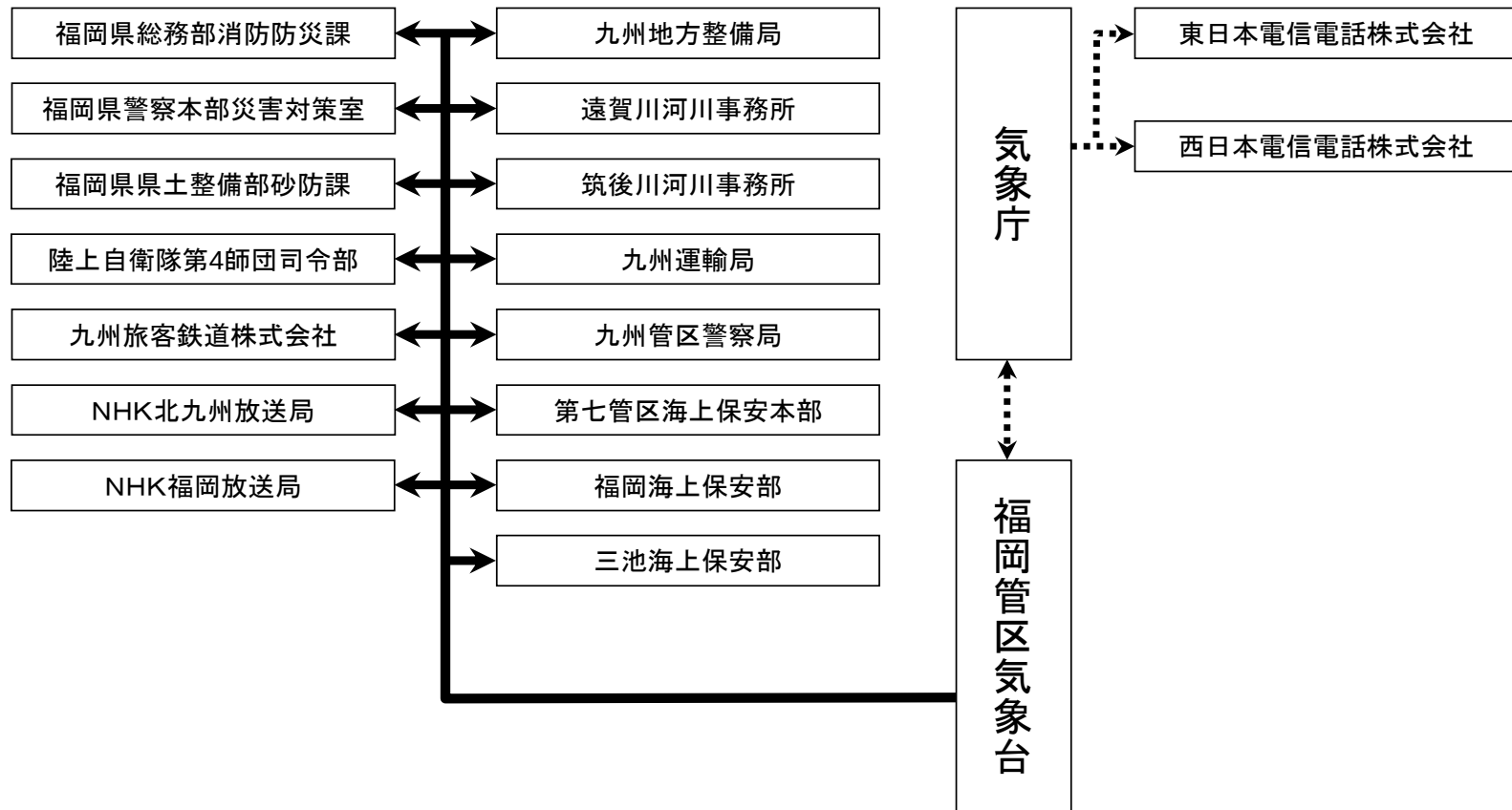
福岡管区気象台気象情報伝送系統図
